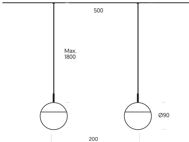
BALO PENDANT
